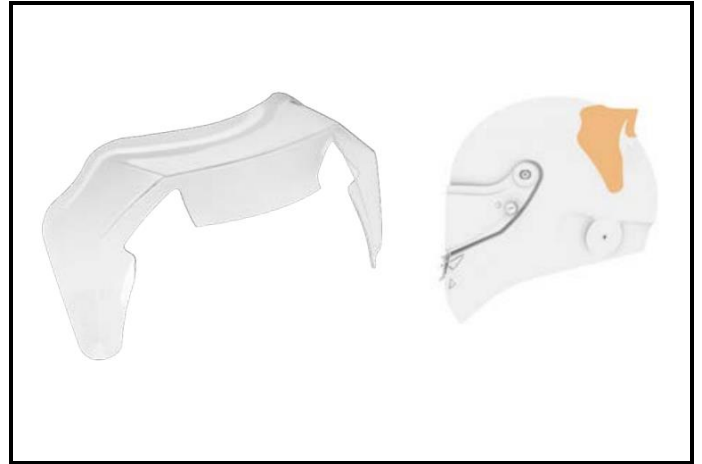
E4) Spoiler RBR24 MK2 (polycarbonate)
