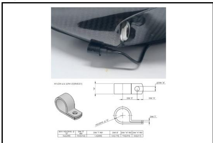
E3) CLIPS SIDE PORT CONNECTOR
