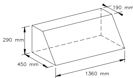
Dessin / Drawing 279-4
