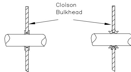
Dessin / Drawing 253-60
