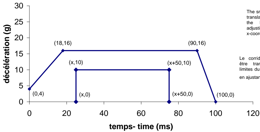
Dessin 7 6 : Corridor de décélération (second impact arrière) Drawing 7 6: Deceleration corridor (second rear impact)
